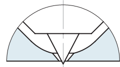
SMF – offene Düse mit Spitze Ausführung „Spitze“ Vorkammer-Ausführung A
