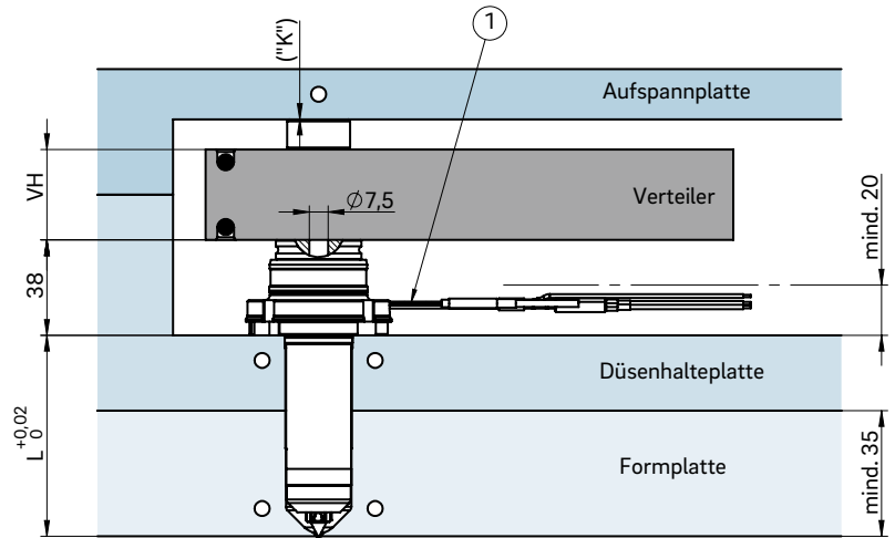
Beispiel Ausnehmung für Düsenkopf, Strom- und Thermofühleranschluss
