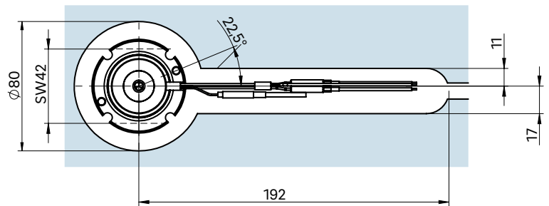
Beispiel Ausnehmung für Düsenkopf, Strom- und Thermofühleranschluss
